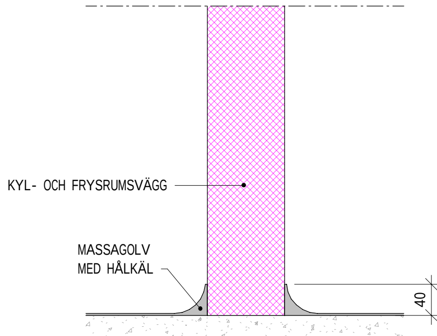
IVD12 - PRINCIPDETALJ MASSAGOLV MOT KYL-/FRYSRUMSVÄGG 1 : 5
