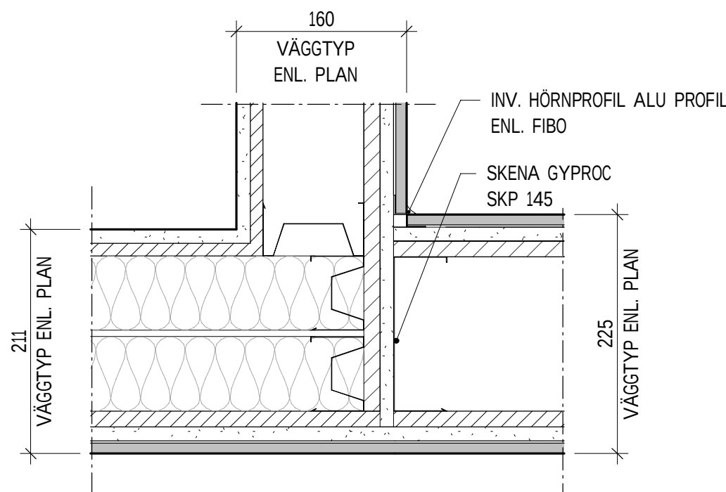
IVD05 - MÖTE 3 VÄGGAR 1 : 5
