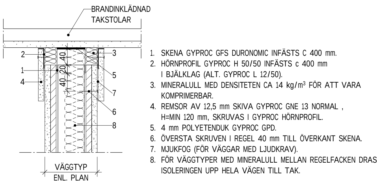
IVD13 - PRINCIPDETALJ TELESKOPANSLUTNING INNERVÄGG 1 : 5
