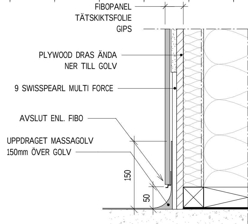
IVD11 - PRINCIPDETALJ MASSAGOLV MOT YTTERVÄGG 1 : 5
