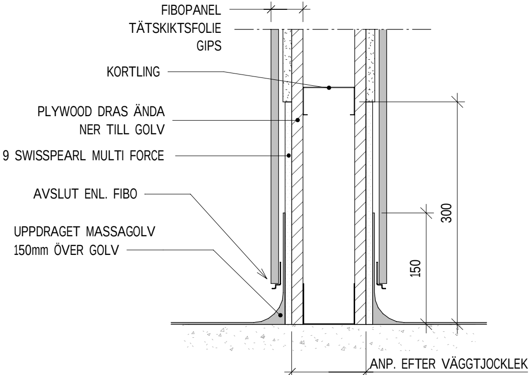
IVD10 - PRINCIPDETALJ MASSAGOLV MOT INNERVÄGG 1 : 5
