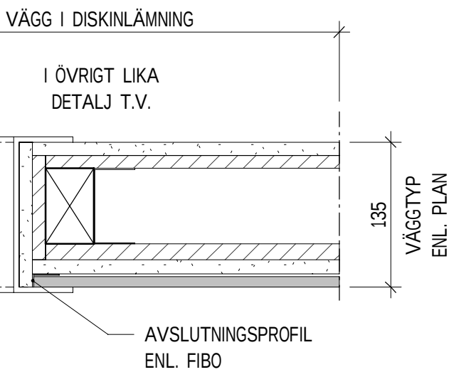
IVD06 - INKLÄDNAD FÖRDELARSKÅP 1 : 5
