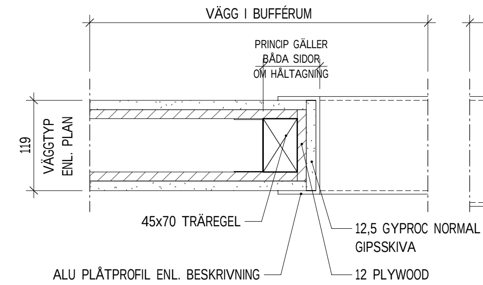
IVD07 - HÅLTAGNING VÄGG 1 : 5
