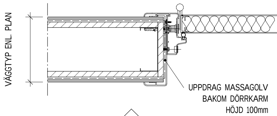
IVD01 - PRINCIPDETALJ MÖTE INNERVÄGG 1 : 5
