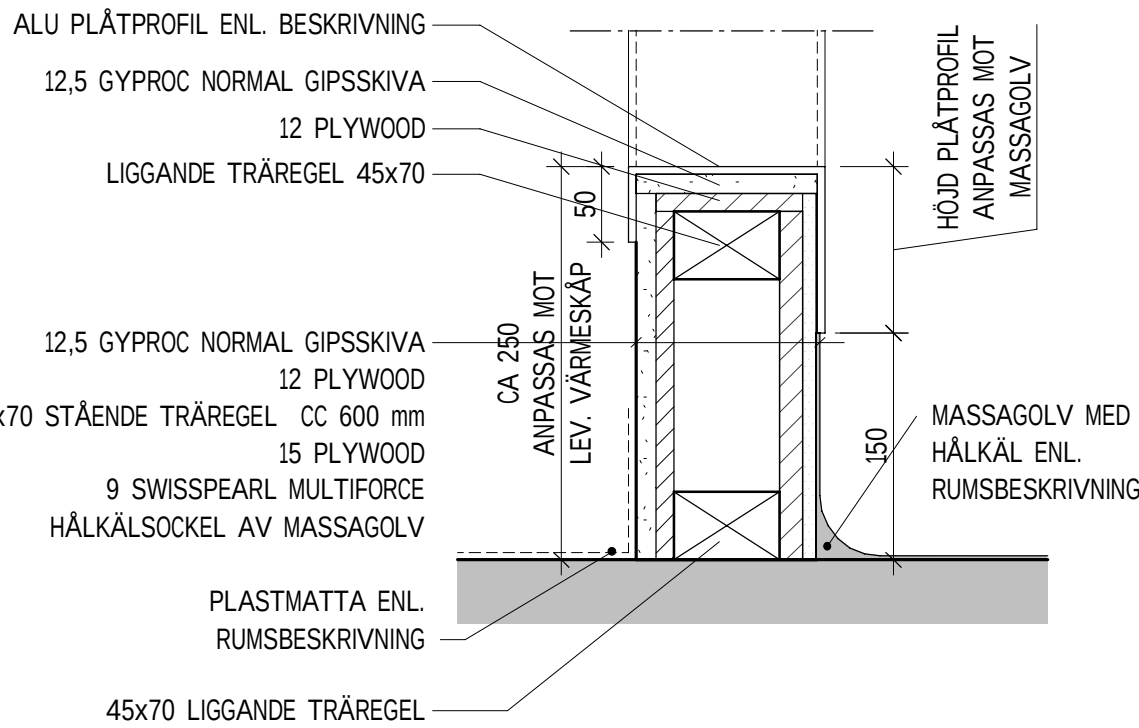
IVD14 - HÅLTAGNING VÄGG VÄRMESKÅP 1 : 5
